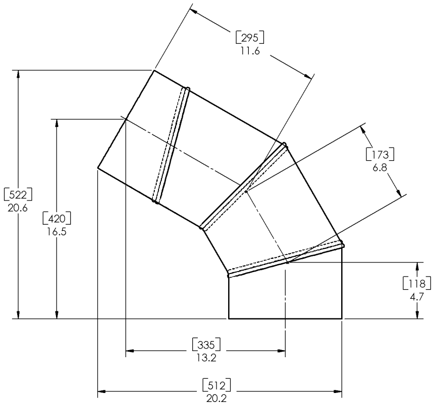
60° ANGLE SCALE 1:1
