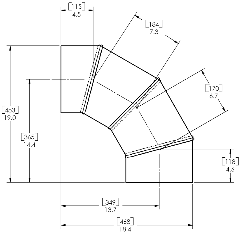
90° ANGLE SCALE 1:1
